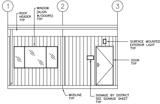
ELEVATION A
