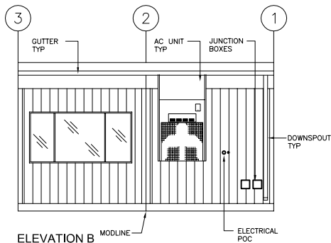
ELEVATION B
