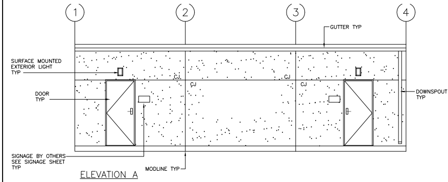
ELEVATION A
